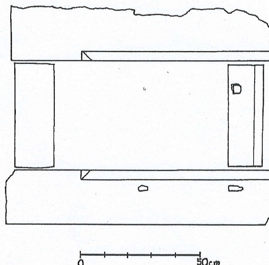
Obr. 7. Nebovidy, tvrz. Ostění okna druhotně sestavené ze starších dílů. Všechny kresby autor. - Nebovidy, Feste: Fensterleibungen - sekundär aus älteren Teilen zusammengesetzt. Alle Zeichnungen: der Autor.
