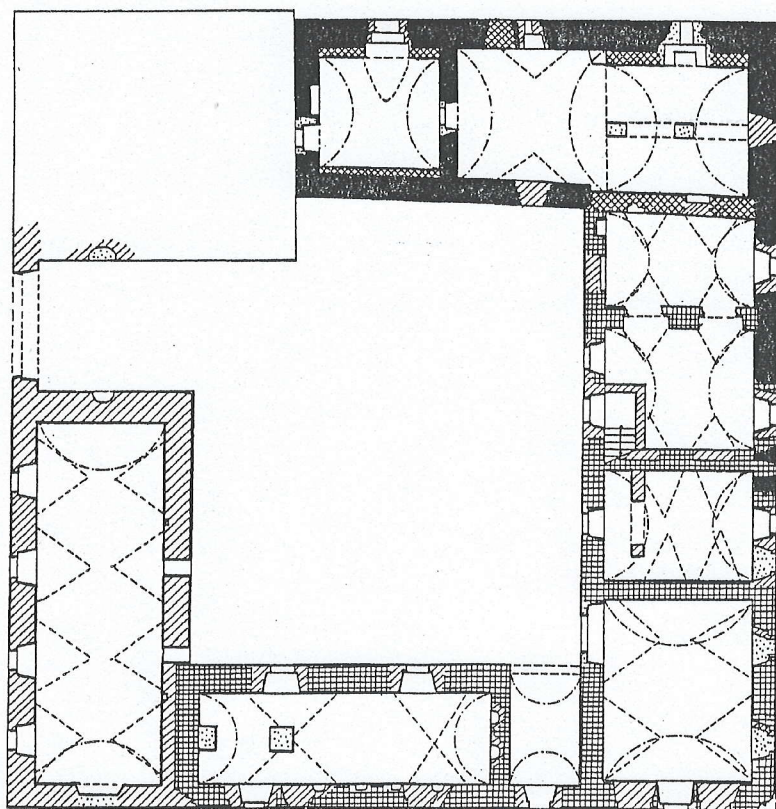
Obr. 3. Nebovidy, tvrz. Půdorys přízemí, měřeno v r. 1984 a 1991. Černě starší gotické, křížem šrafované mladší gotické zdivo, křížem kolmo k obrysu šrafované renesanční, šrafované barokní, tečkované mladší. - Nebovidy-Feste: Grundriß des Erdgeschosses, vermessen im J. 1984 und 1991. Älteres gotisches Mauerwerk schwarz, jüngeres gotisches Mauerwerk gekreuzt schraffiert, senkrecht zum Umriß schraffiert das Renaissance-Mauerwerk, schraffiert das barocke und punktiert das jüngere Mauerwerk.
