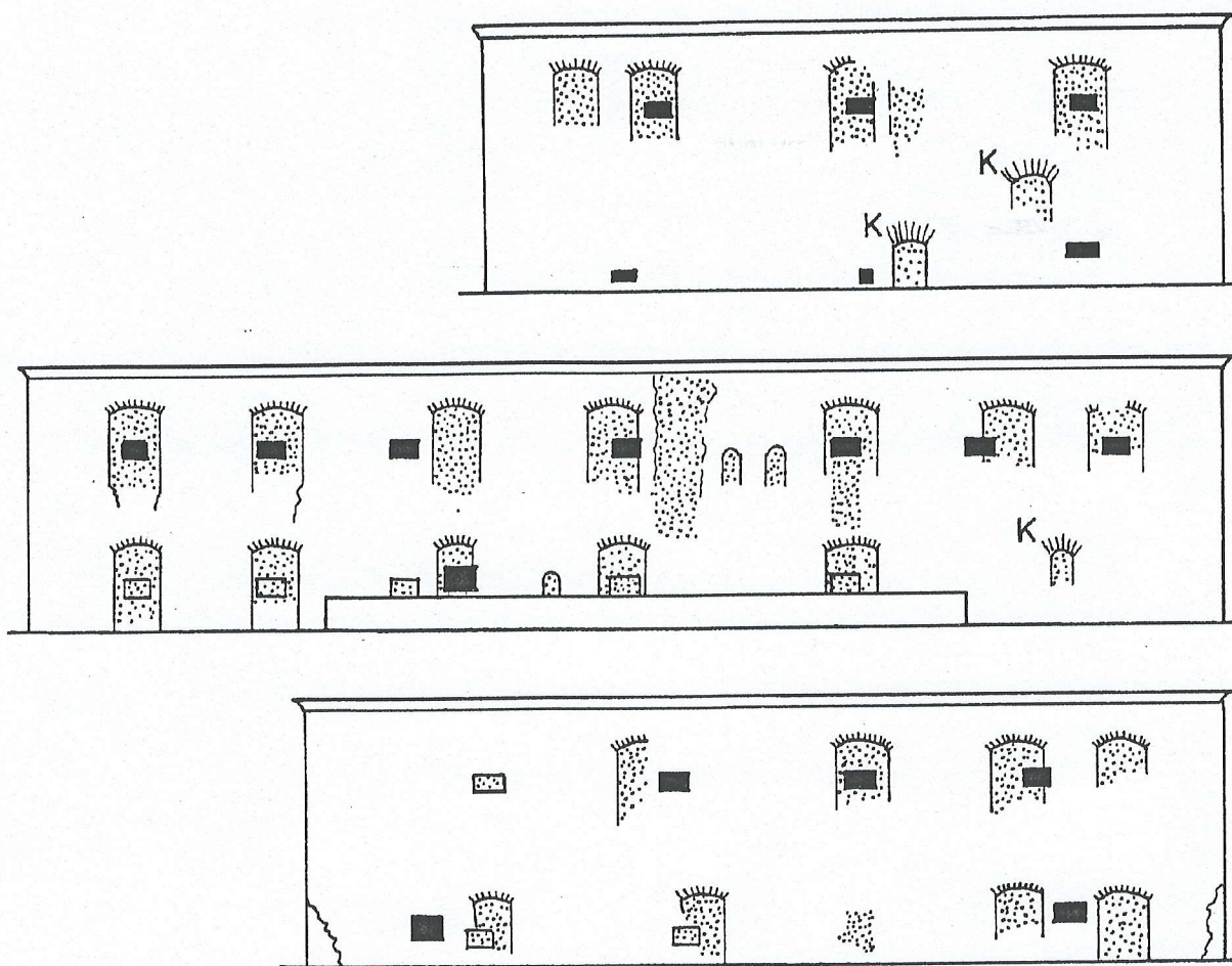
Obr. 5. Nebovídky, tvrz. Schematické pohledy na průčelí s vyznačením zazděných otvorů. Shora východní, jižní a západní průčelí. Tečkovaně zazdívký a větší cihelné vysprávky, záklenky z lomového kamene označeny písmenem K. - Nebovídky-Feste: Schematische Ansichten der Fassade mit Andeutungen der vermauerten Öffnungen. Oben die östliche, südliche und westliche Fassade. Punktiert die Vermauerungen und größeren Reparaturen mit Ziegeln, die Fensterbögen aus Bruchstein mit K bezeichnet.
